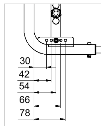
Schwerpunkt Seitenansicht
